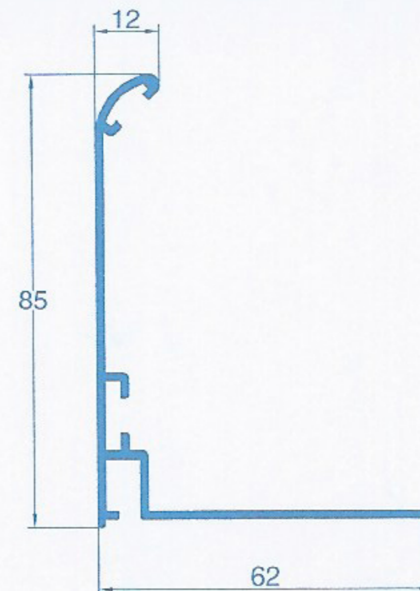
SOLAPE DECORATIVO
